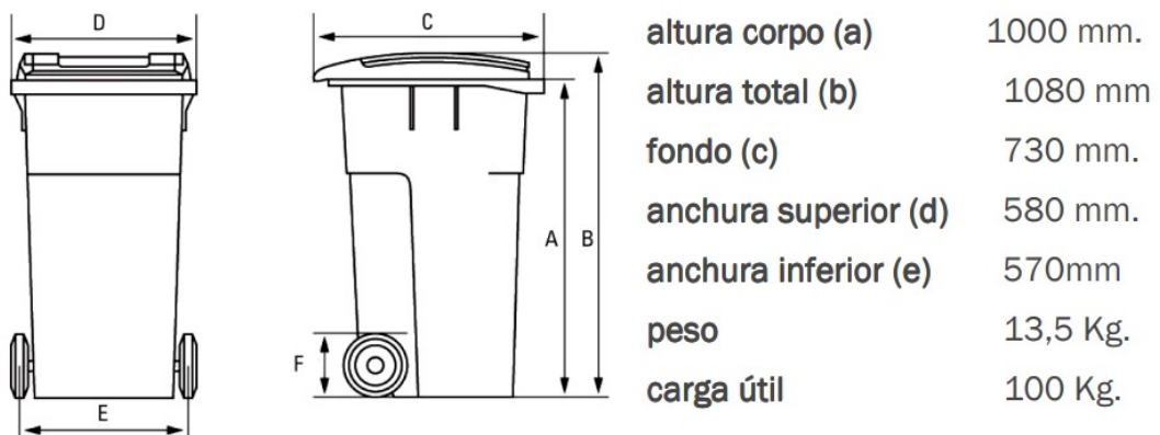
Figura 2. Detalle das dimensións do contedor
